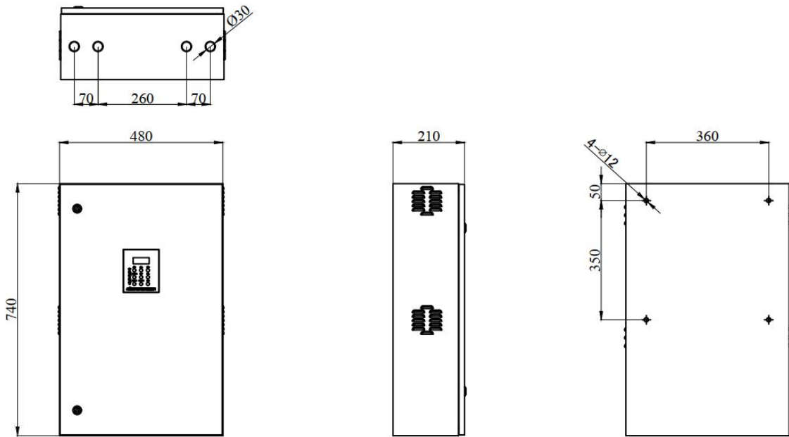
图 2.1 外形尺寸图
